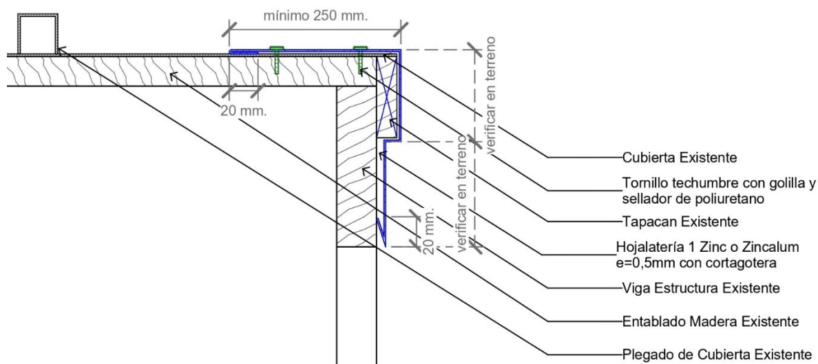
Corte Detalle Hojalaterías alero lateral oriente.
