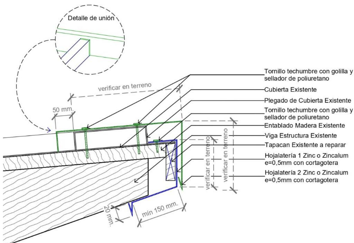
Corte Detalle Hojalaterías alero superior sur.
